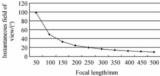
图 6 瞬时视场与焦距关系曲线
