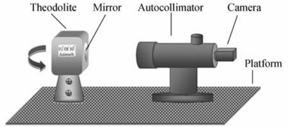
图 8 光斑图像配准实验装置
